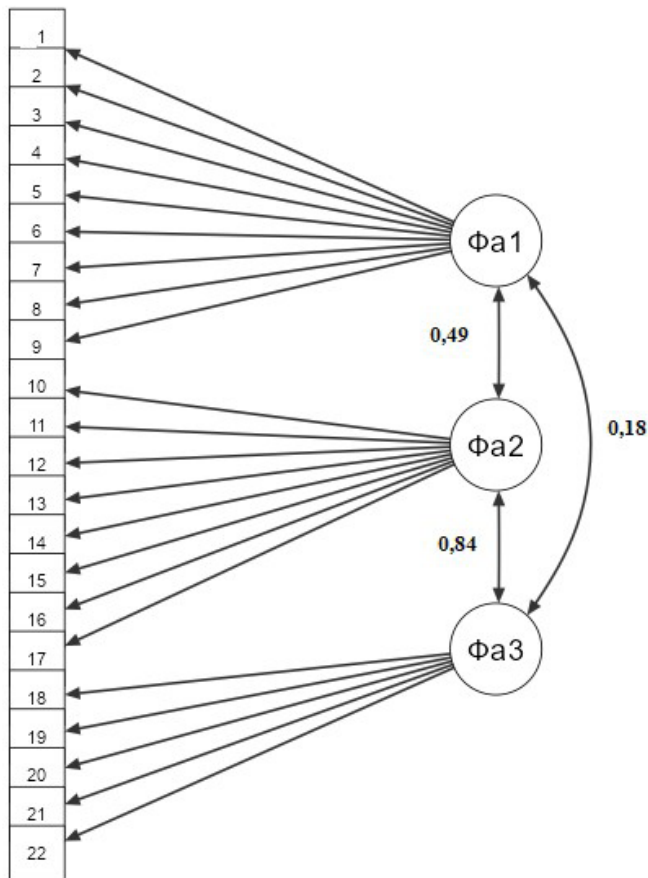
Рис. 2 / Fig. 2. Конфирматорный факторный анализ GSBP (Общей шкалы воспринимаемого фаббинга): Фа1 – воспринимаемые нормы; Фа2 – чувство игнорирования; Фа3 – межличностный конфликт (фабб) / Confirmatory factor analysis of the GSBP (Generic Scale of Being Phubbed): Fa1 – perceived norms; Fa2 – feeling ignored; Fa3 – interpersonal conflict (phubby)
